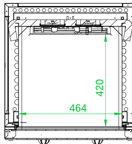
SEZIONE A-A
