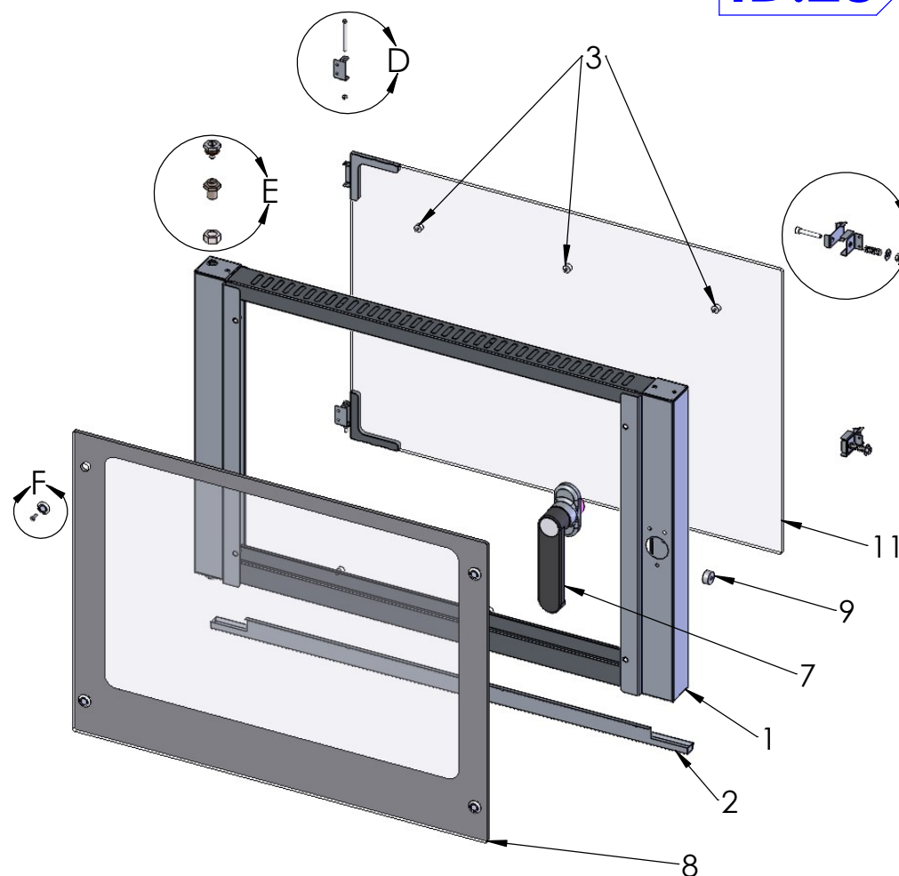
DETTAGLIO E kit perno porta
