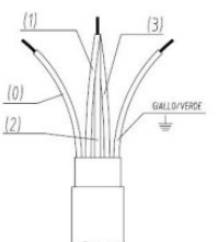
V220-240/2 SINGLE-PHASE 단일 위상 CONNECTION 연결
