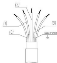
V380-415/3+N THREE-PHASE 삼상 별 CONNECTION WITH NEUTRAL 중성과의 연결
