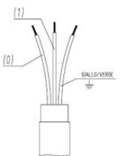
V220-240/2 SINGLE-PHASE 단일 위상 CONNECTION 연결
