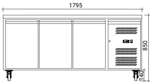
XUB6C18S3V / XUB6F18S3V
