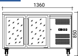
XUB7C13G2V
