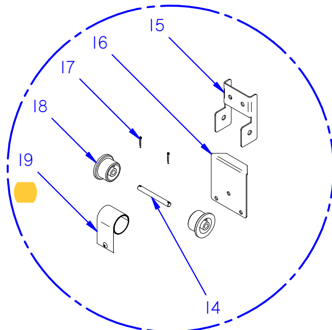
DETALLE A
