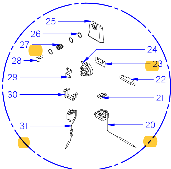
DETALLE B
