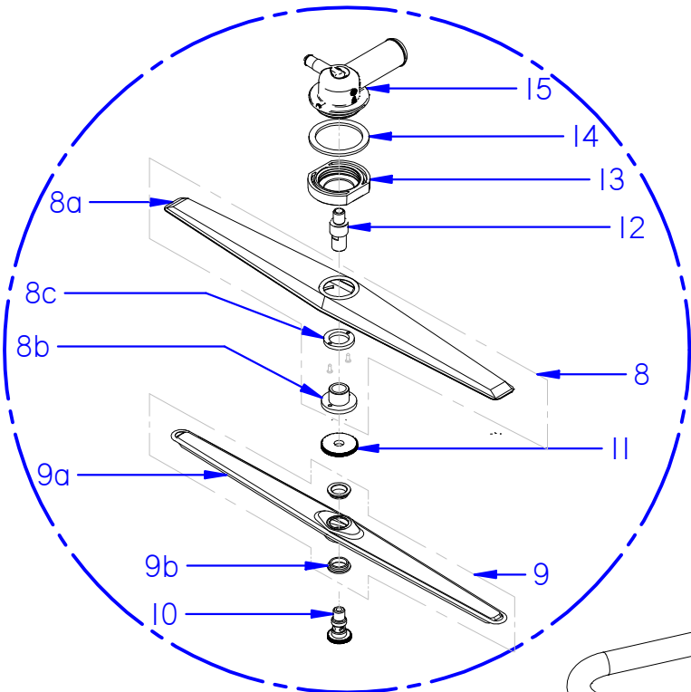
DETALLE A
