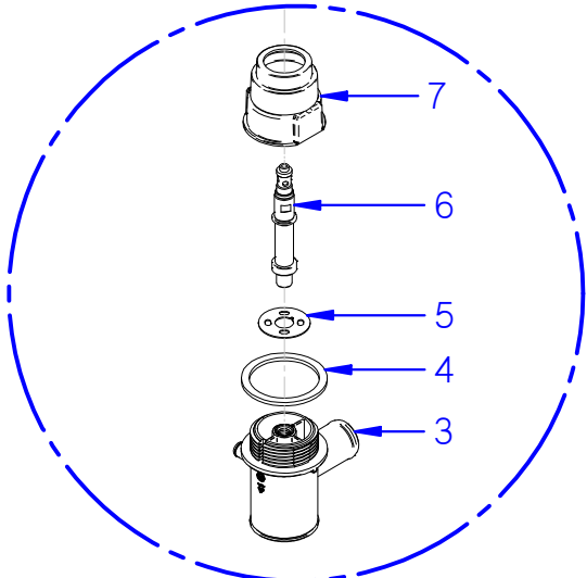
DETALLE B
