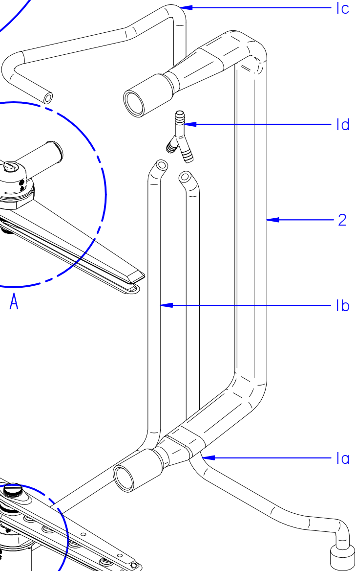
DETALLE B
