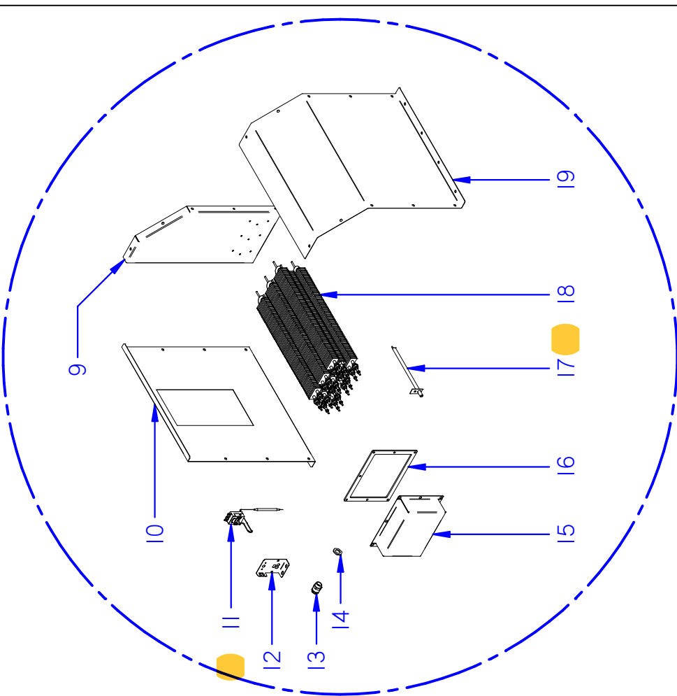
DETALLE A
