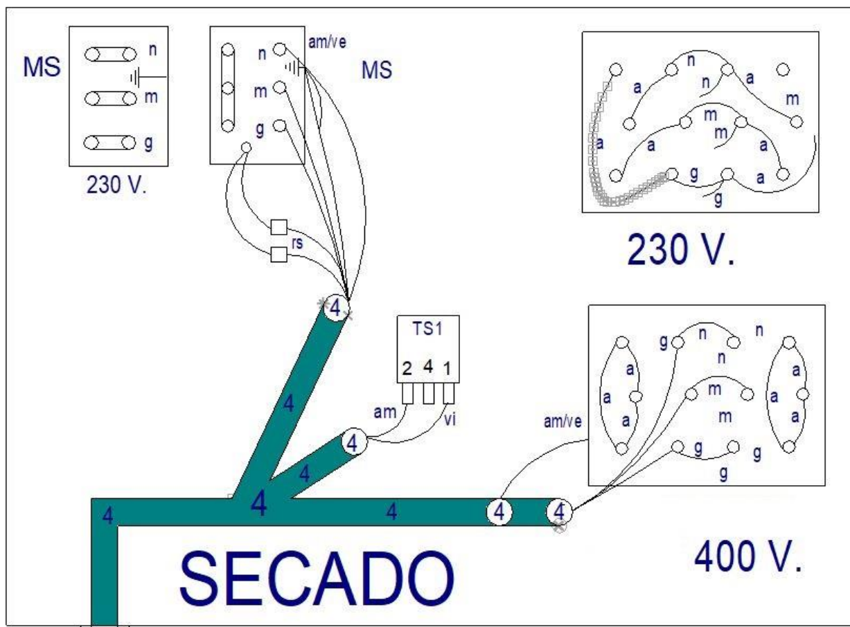
Imagen 12.- Instalación en el túnel de secado
