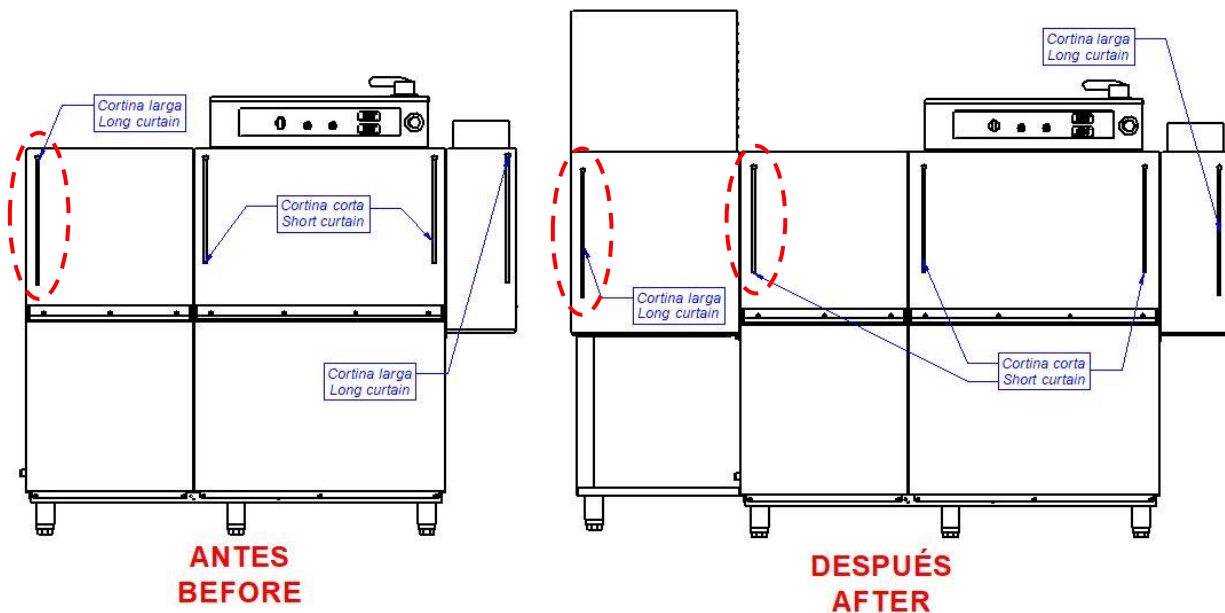
Imagen 10.- Colocar cortinas
