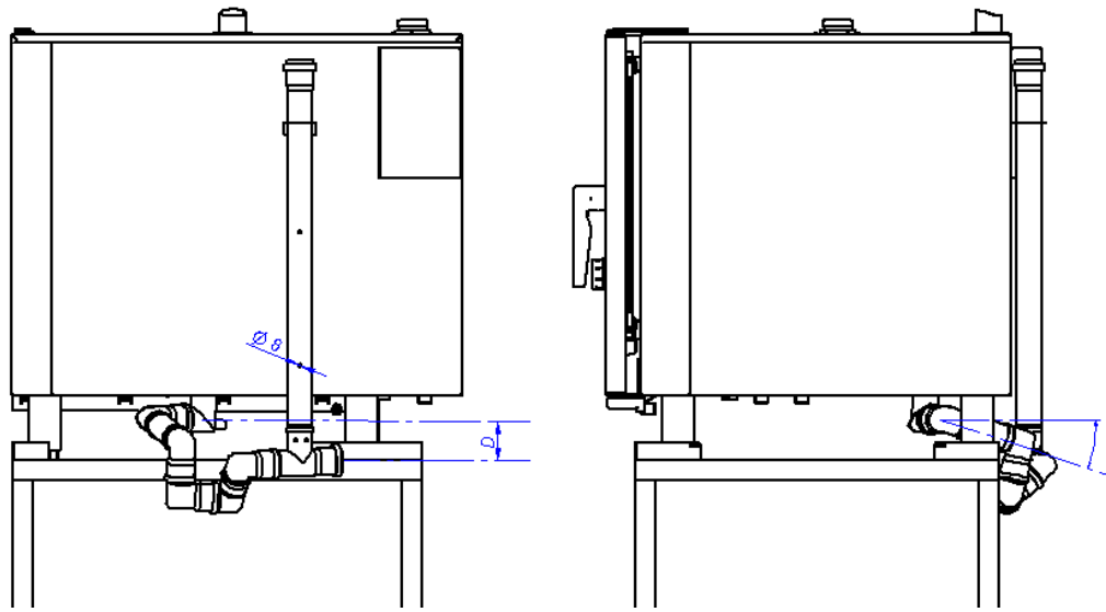
图 13: 台式机型号 061-101-102
