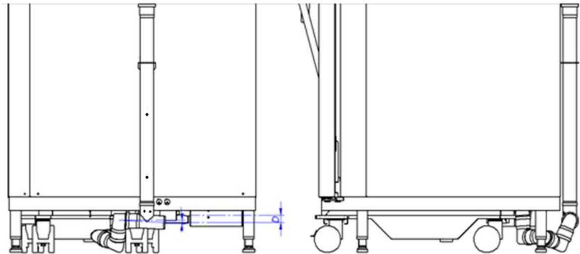
图 14: 落地型 201 和 202 型
