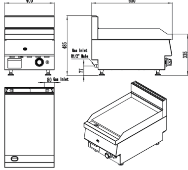
AT65G4G-C
