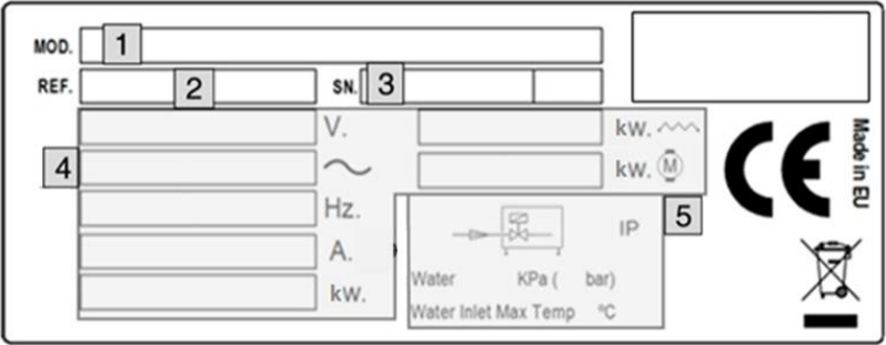
PLAQUE SIGNALÉTIQUE
