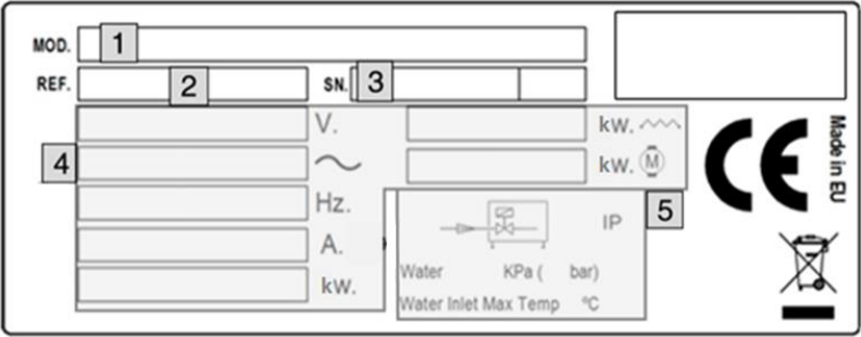
TABLICZKA ZNAMIONOWA
