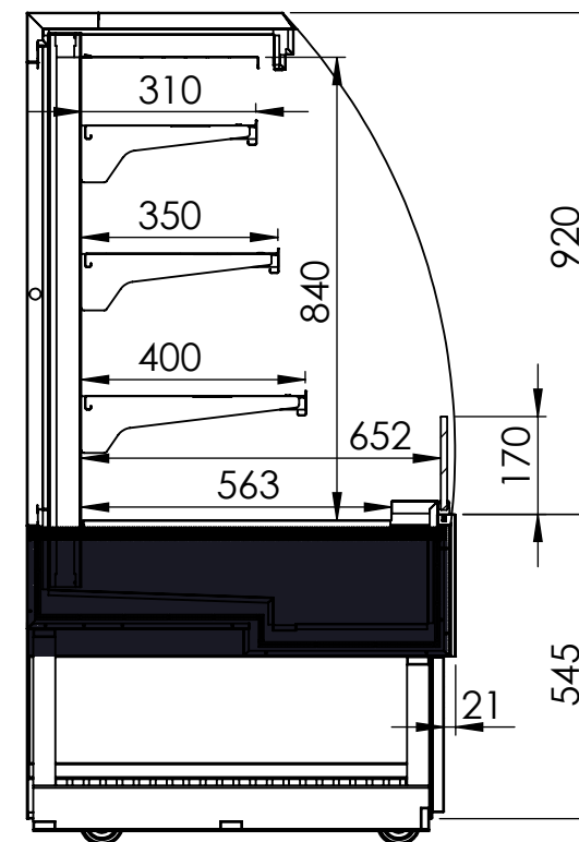
SEZIONE C-C
