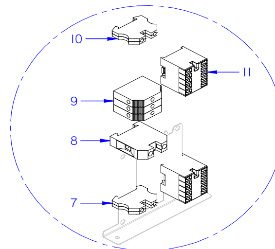
DETALLE A
