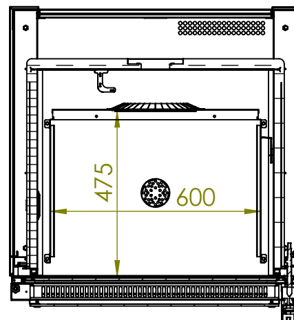
SEZIONE F-F
