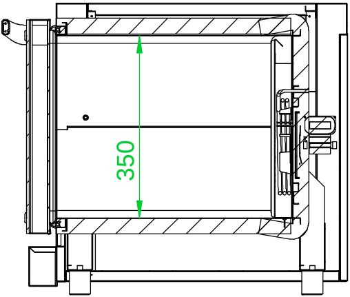
SEZIONE B-B
