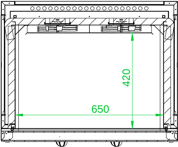
SEZIONE A-A
