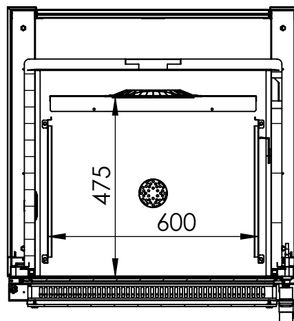
SEZIONE D-D
