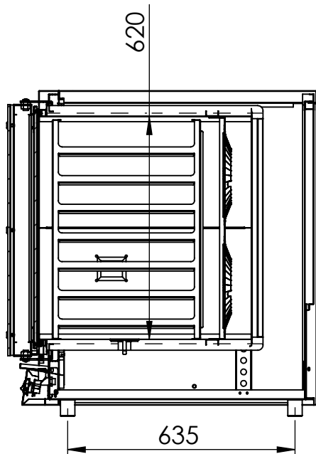
SEZIONE C-C
