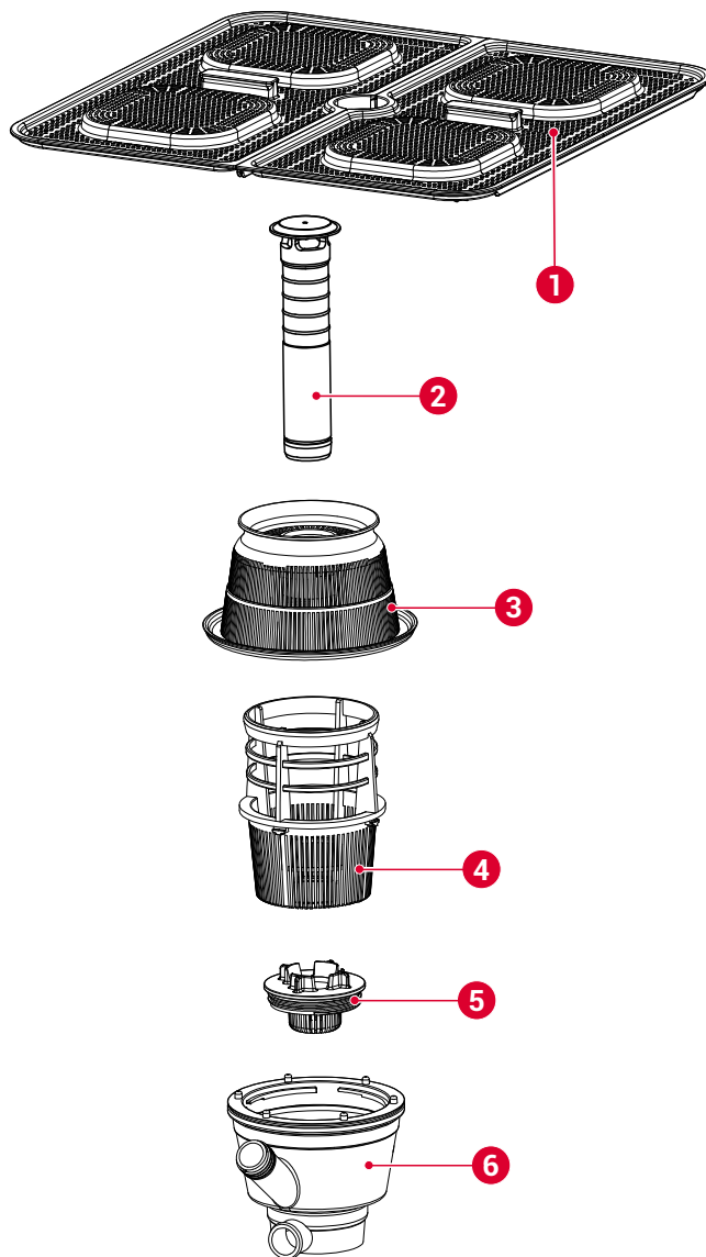
Abb. 4: Maschinenfilter
