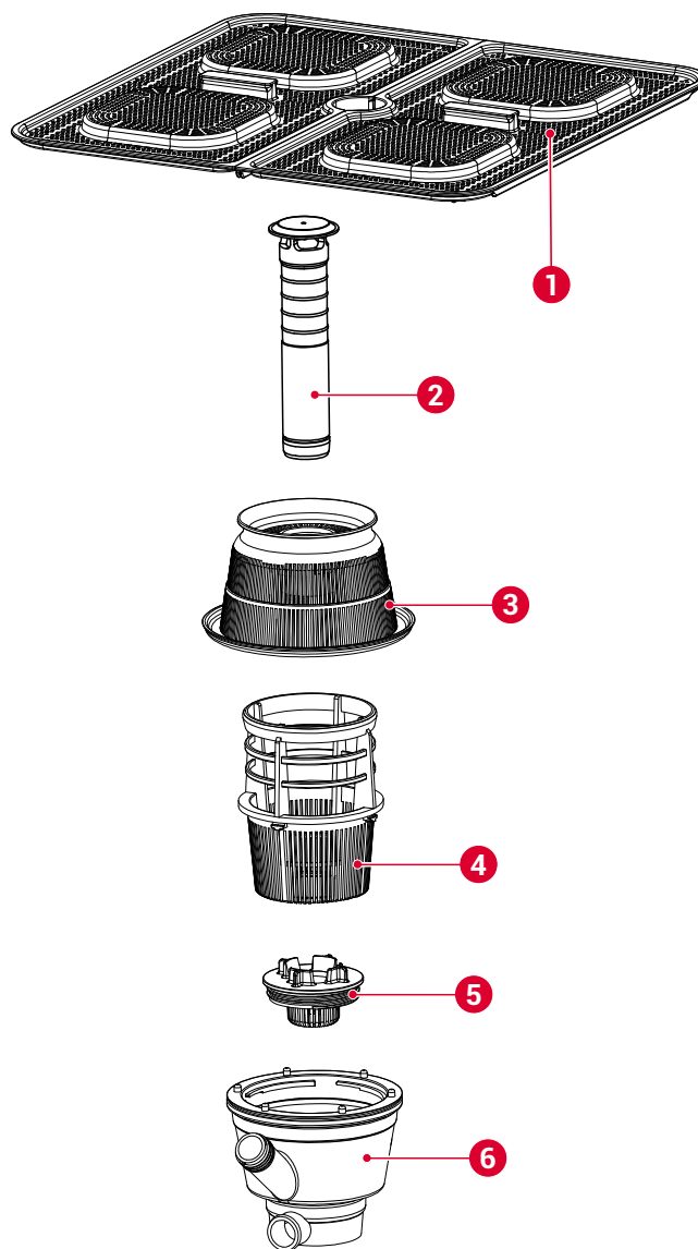
Abb. 4: Maschinenfilter
