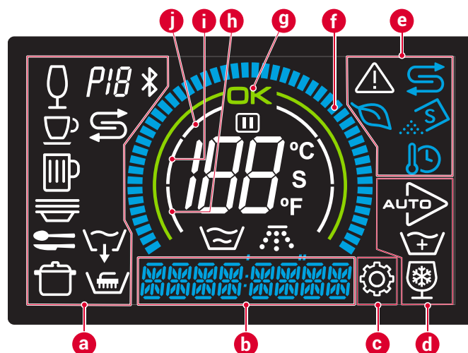
Abb. 3: LCD-Display
