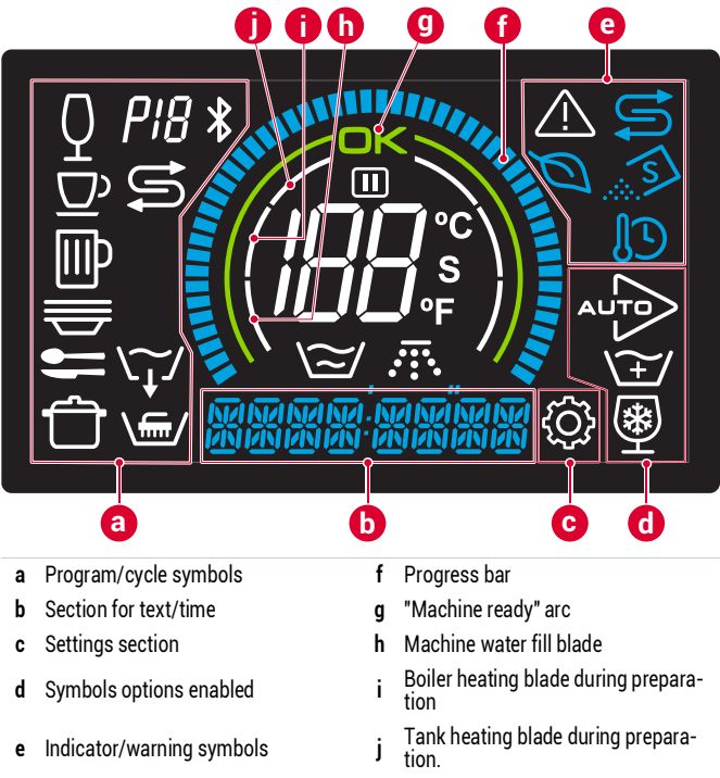
Fig. 3: LCD Display
