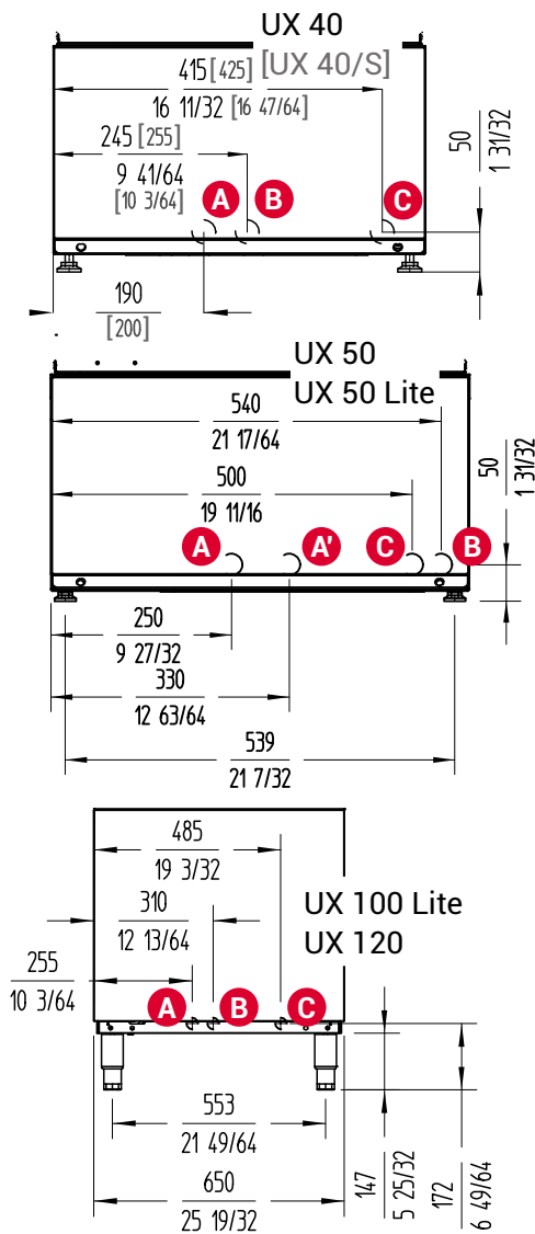
Abb. 1: Maschinenanschlusspunkte
