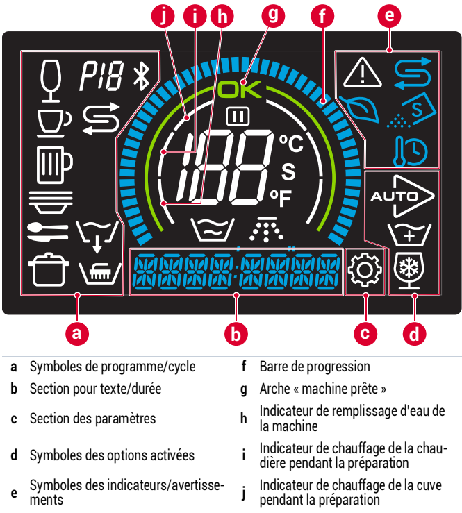
Fig. 3: Écran LCD
