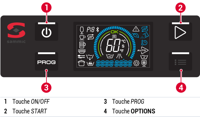
Fig. 2: Panneau de commande et touches à LED
