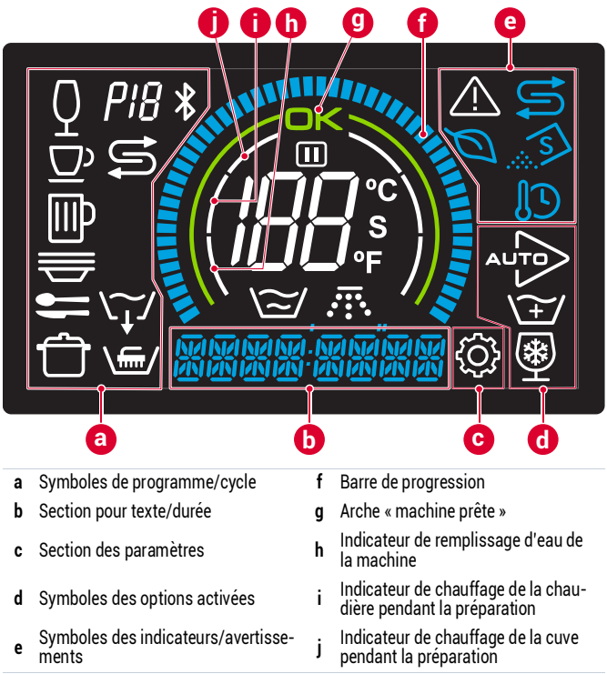
Fig. 3: Écran LCD
