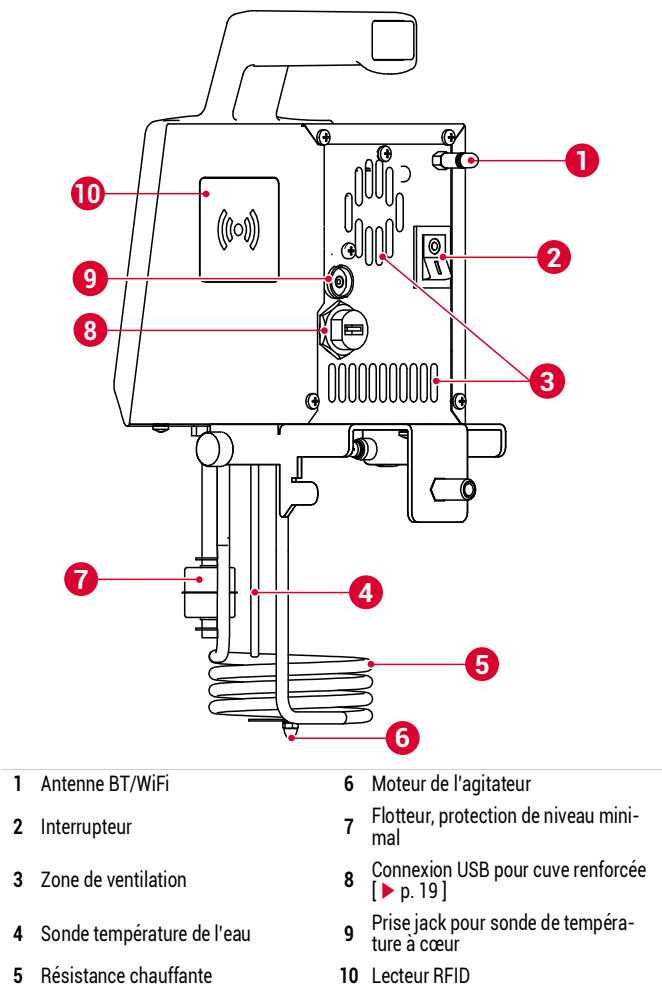
Fig. 1: SmartVide X/XL, principaux composants, partie 1
