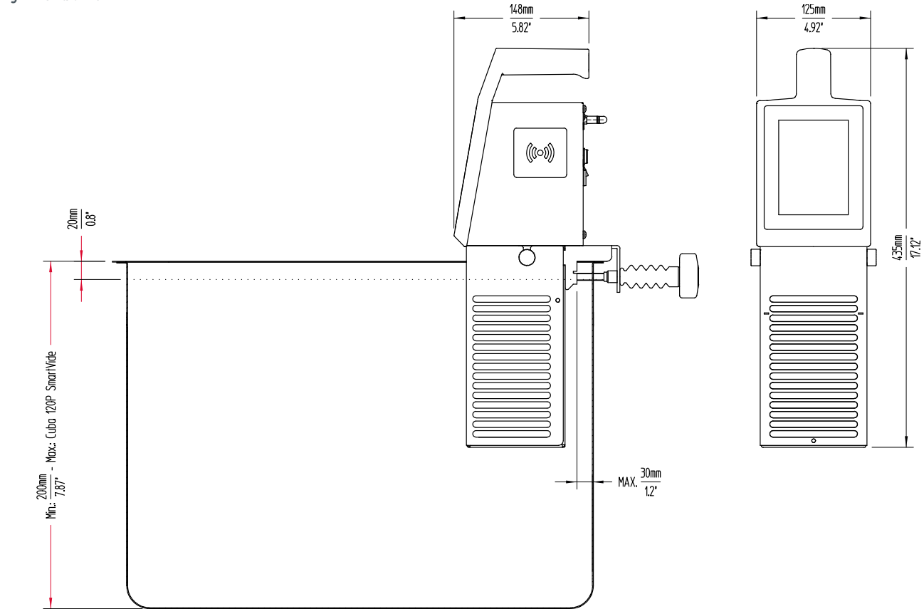
Fig. B: SmartVide XL
