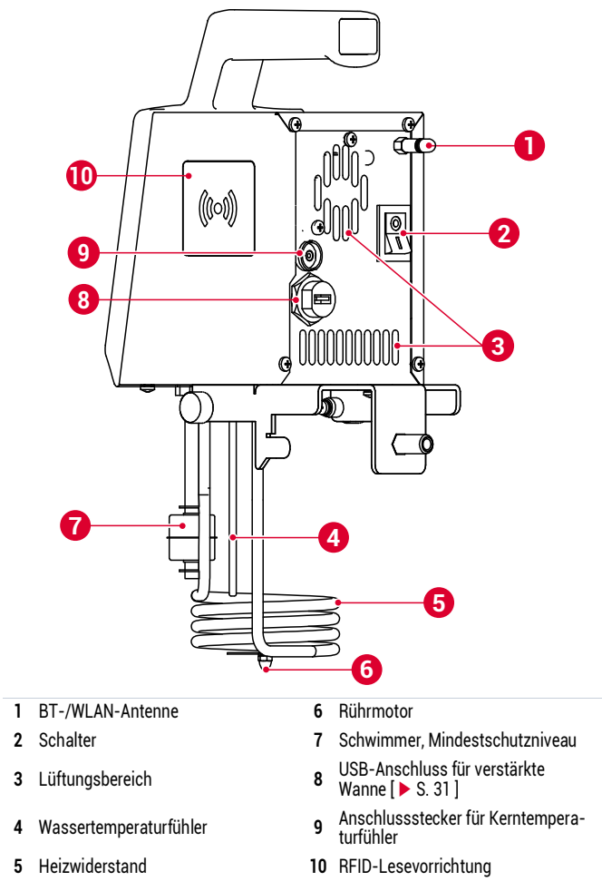
Abb. 1: SmartVide X/XL, Hauptkomponenten, Teil 1
