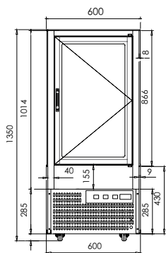
SF820V
