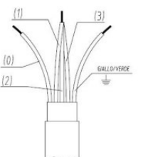
V220-240/2 SINGLE-PHASE 단일 위상 CONNECTION 연결
