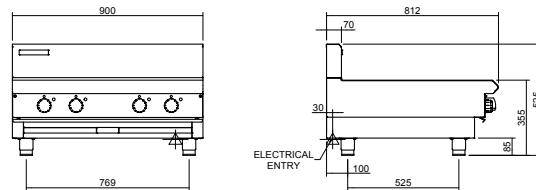
IN514-LS
