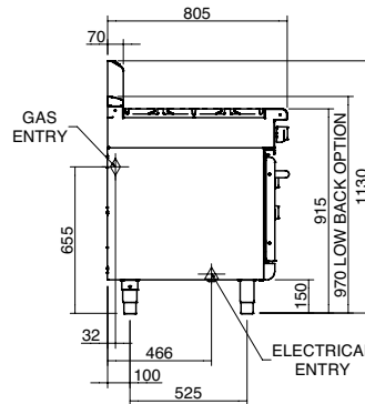
RN8513GE
