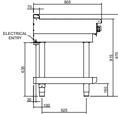
INLB8400R3 / INLB8400R5
