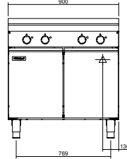
INLB8400R3 / INLB8400R5
