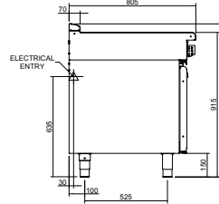
INLB8400R3 / INLB8400R5
