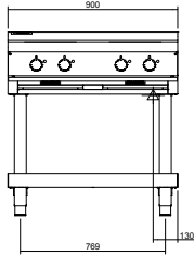
INLB8400-LS
