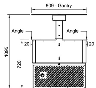
End Elevation
