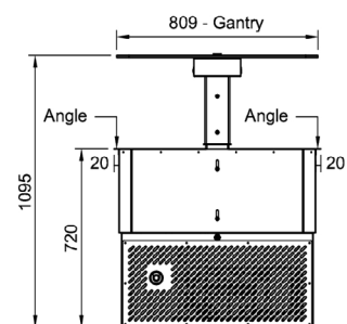
End Elevation
