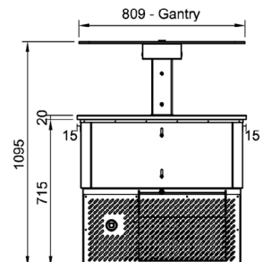
End Elevation
