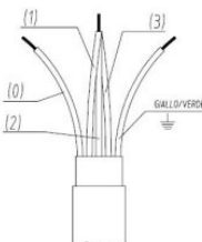
V220-240/2 SINGLE-PHASE 단일 위상 CONNECTION 연결
