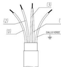
V220-240/3 THREE-PHASE 삼상 델타 CONNECTION 연결
