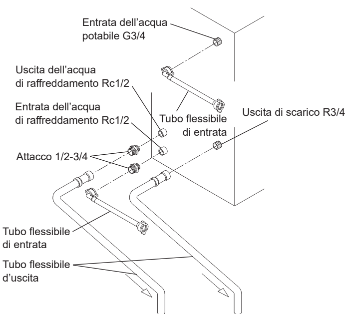
Modello raffreddato ad acqua [b] (IM-45WNE/65WNE)
