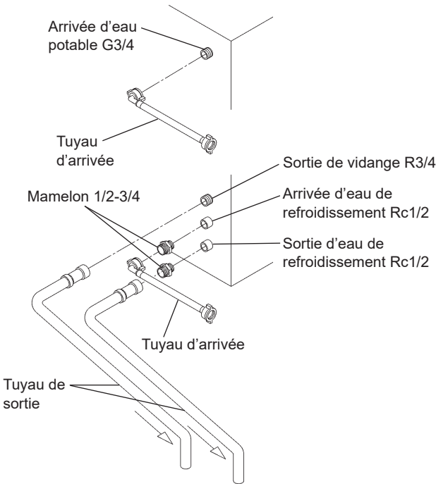
Modèle avec refroidissement par eau [b] (IM-30CWNE/100WNE/130WNE/240WNE)
