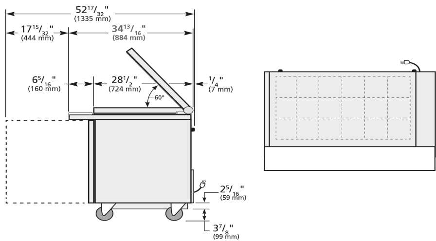
ELEVATION
