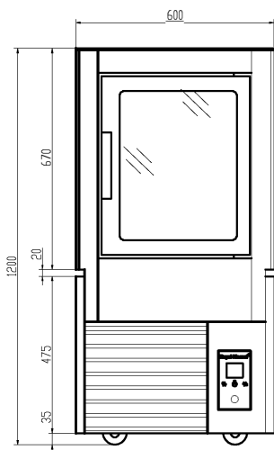
BACK 后视图
