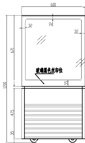
FRONT 前视图
